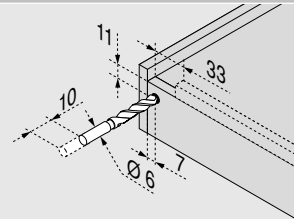
Použite vrtaciu šablónu T65.1000.02
