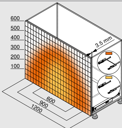
Príklad pre 560F – 30 kg, menovitá dĺžka NL 500 mm, štvorstranná zásuvka, so synchronizáciou
