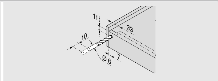
Použite vrtaciu šablónu T65.1000.02
