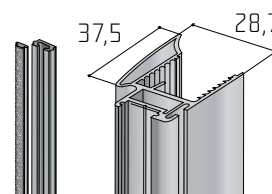
Profil S11N a krycí profil
