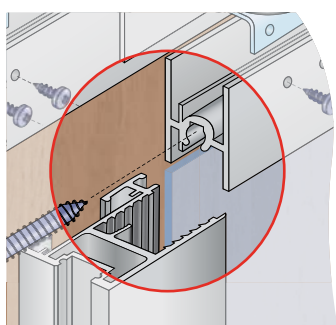
Ověrní výplň: zrcadlo 4 mm nebo bezpečnostní sklo 4 mm
