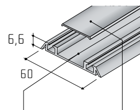
Profil S06 N krycí Profil S06 NN
