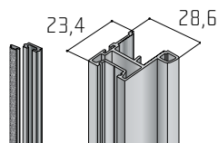
Profil S24
