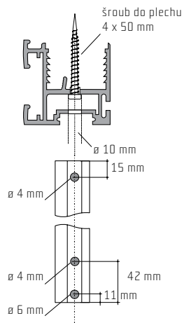
Profil S19
