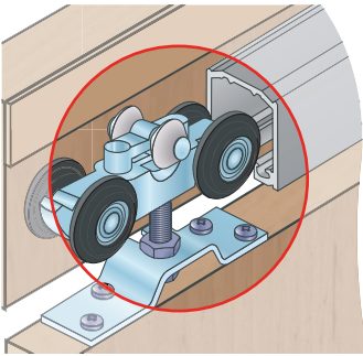
Montáž horního vozíku
