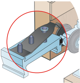
Brzda s tlumičem
